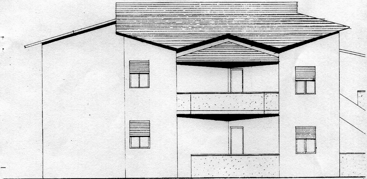
PROSPETTO OVEST.
