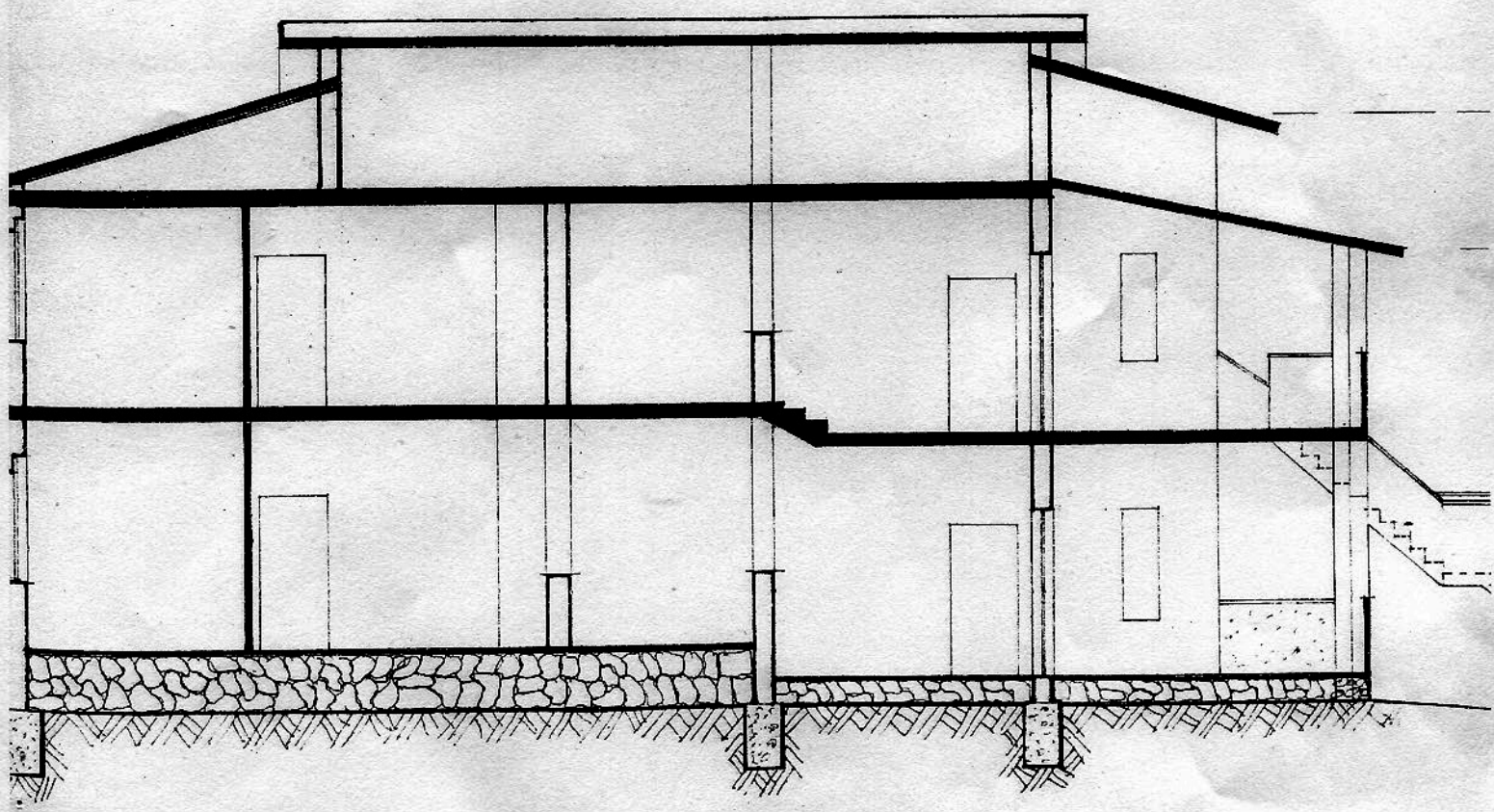
SEZIONE B-B
