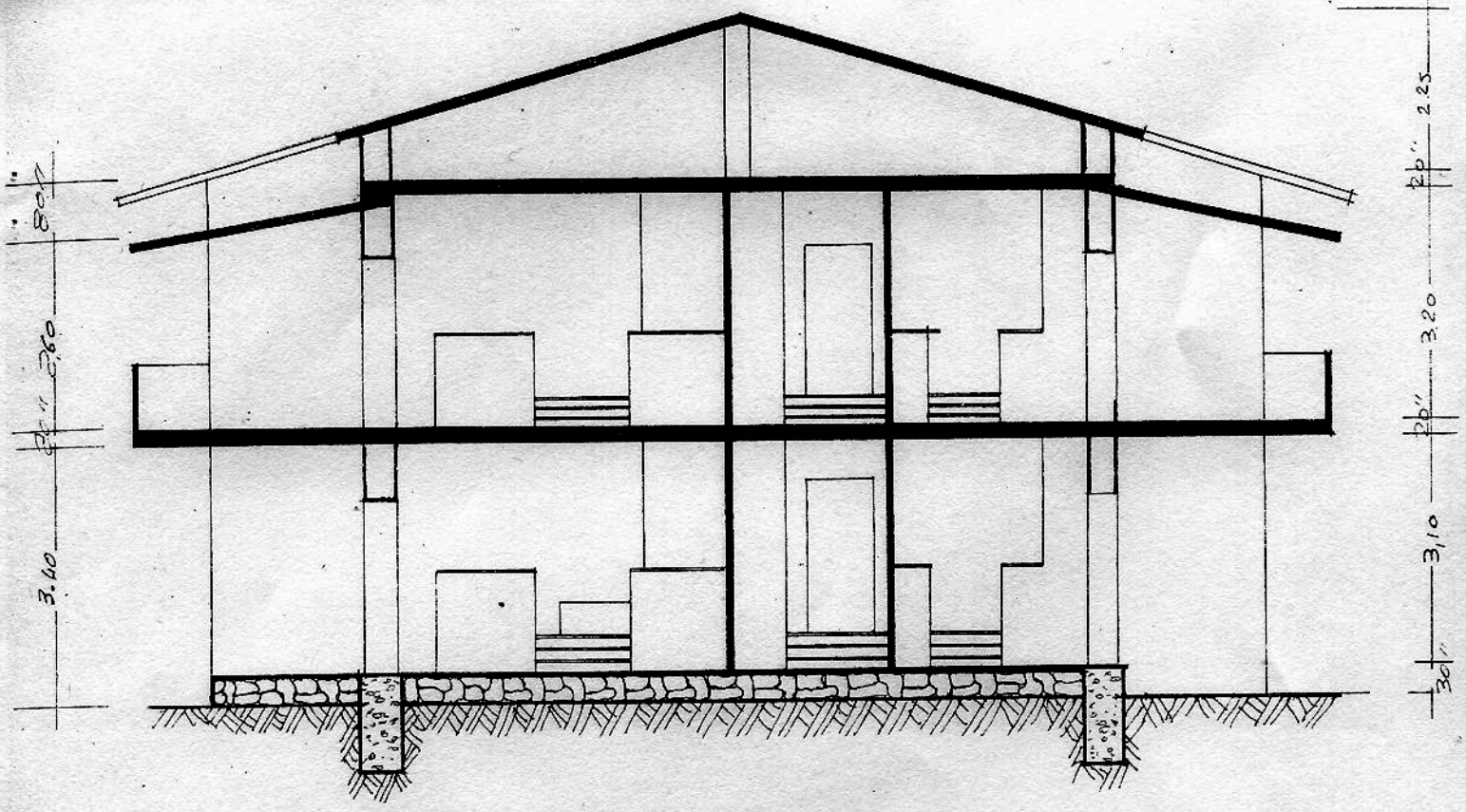
SEZIONE A-A
