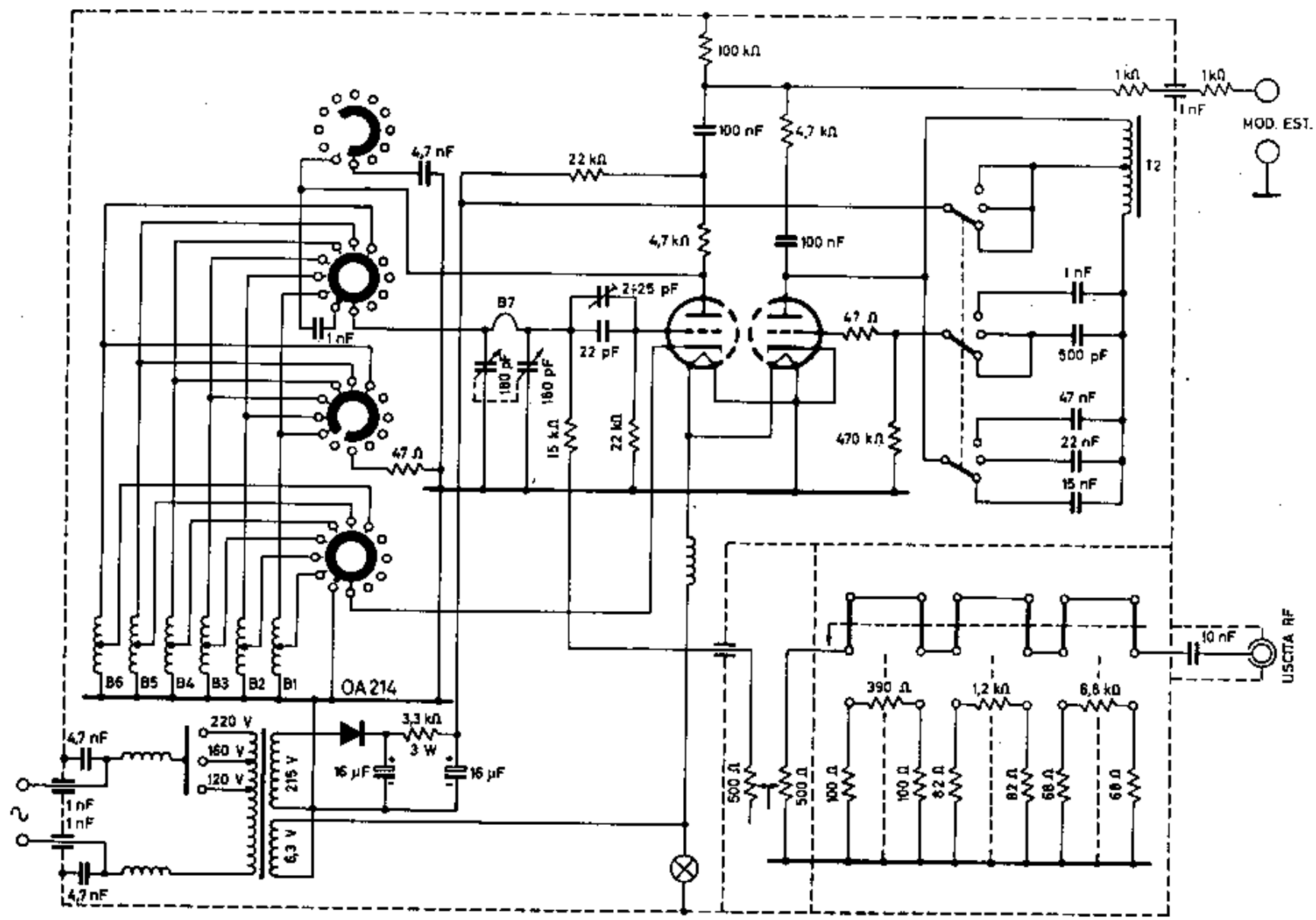
GENERATORE DI SEGNALI UNA MOD. EP 45
