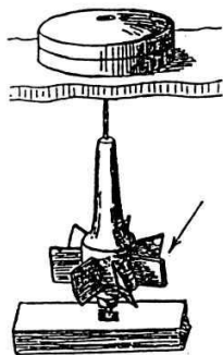
Mulino idraulico "orizzontale."
