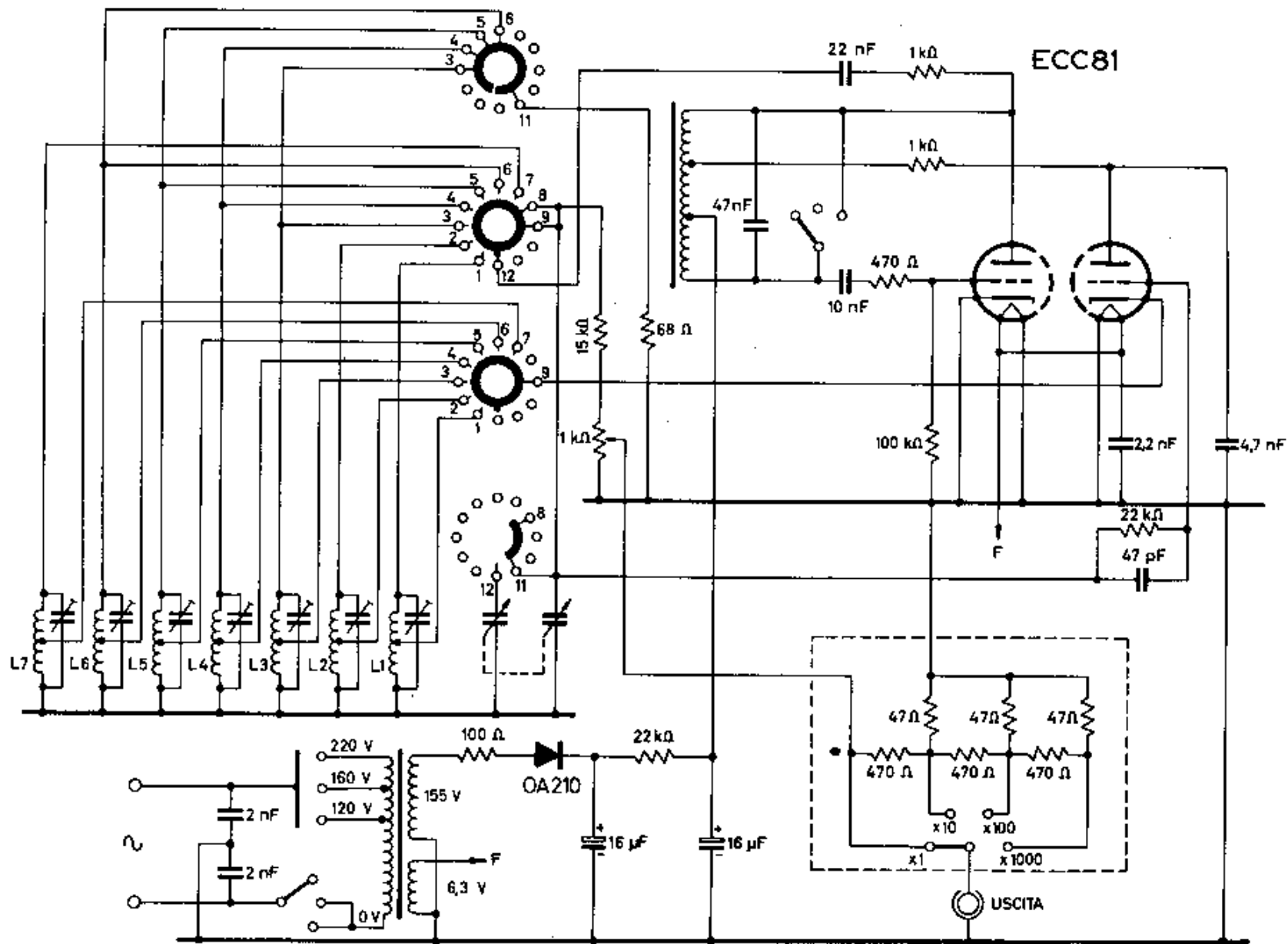
GENERATORE DI SEGNALI UNA MOD. EP 57
