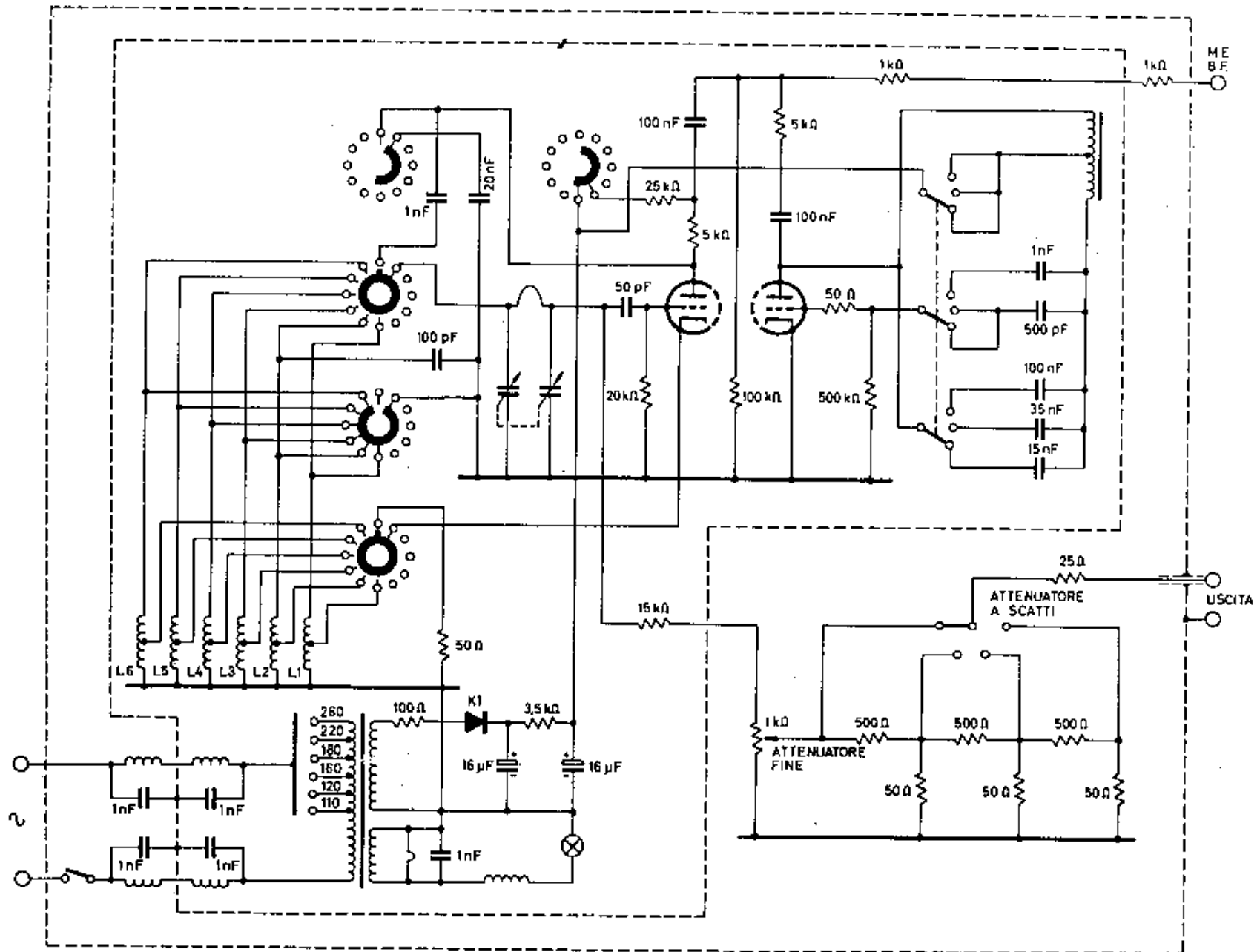
OSCILLATORE MODULATO MECRONIC MOD. 45/S
