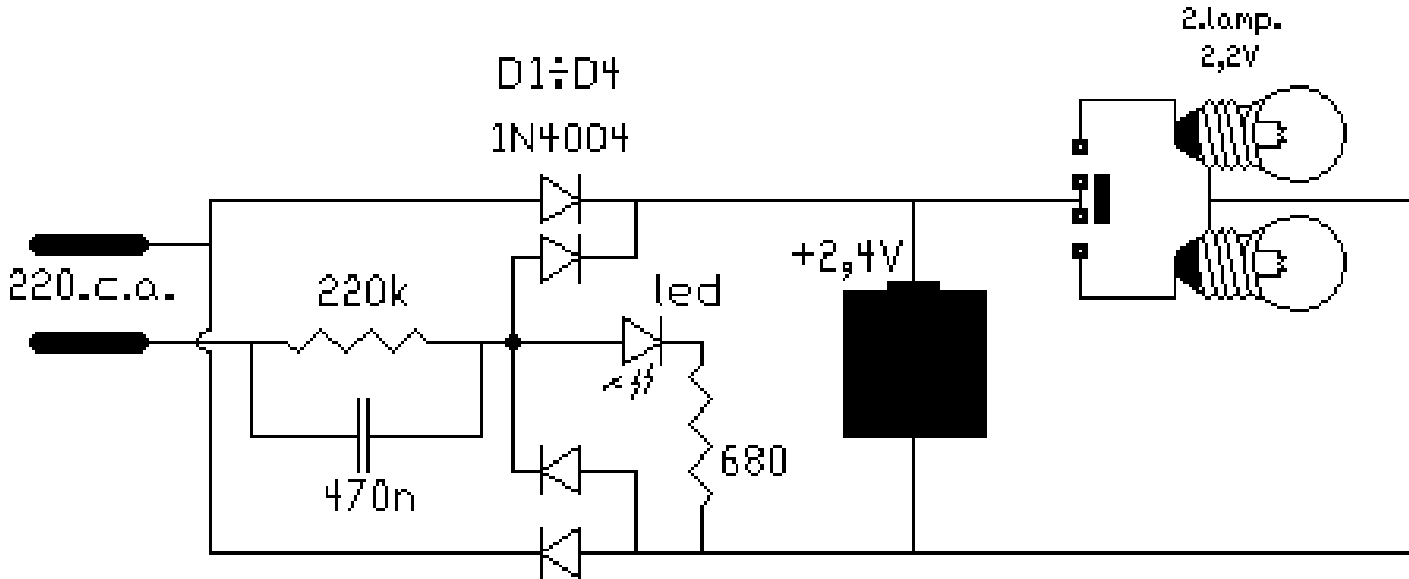
Lampada tascabile ricaricabile ( LINA )
