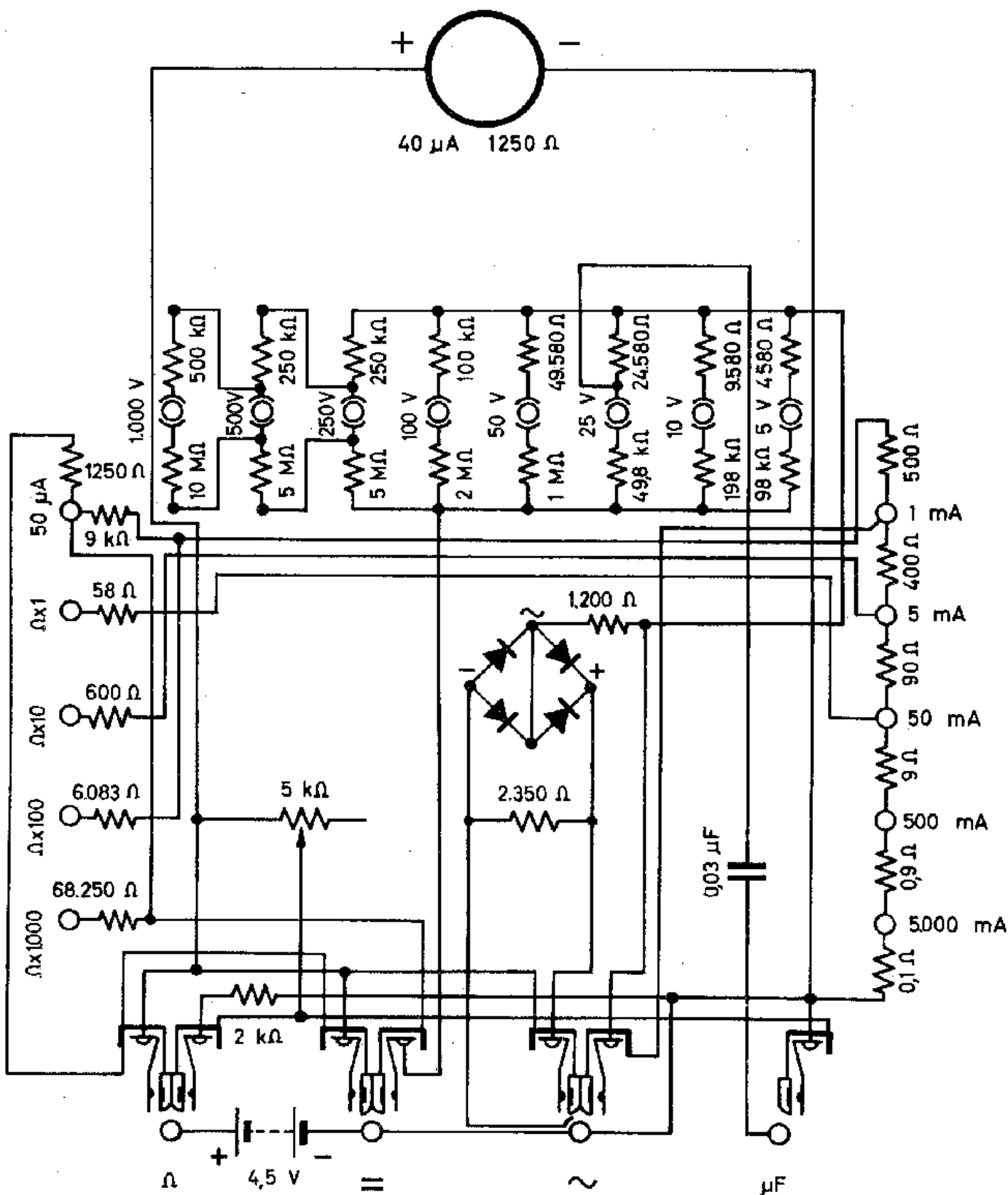
SCHEMA ELETTRICO DELL'ANALIZZATORE ICE MOD.620
