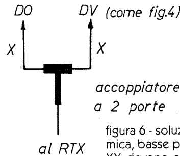
figura 5 - Commutazione di polarizzazioni con schema di comando remoto. I cavi denominati XX, YY e ZZ devono essere a coppie uguali e possibilmente \lambda/2 \cdot V_8 multipli interi. I relè sono a riposo (posizione 1).
