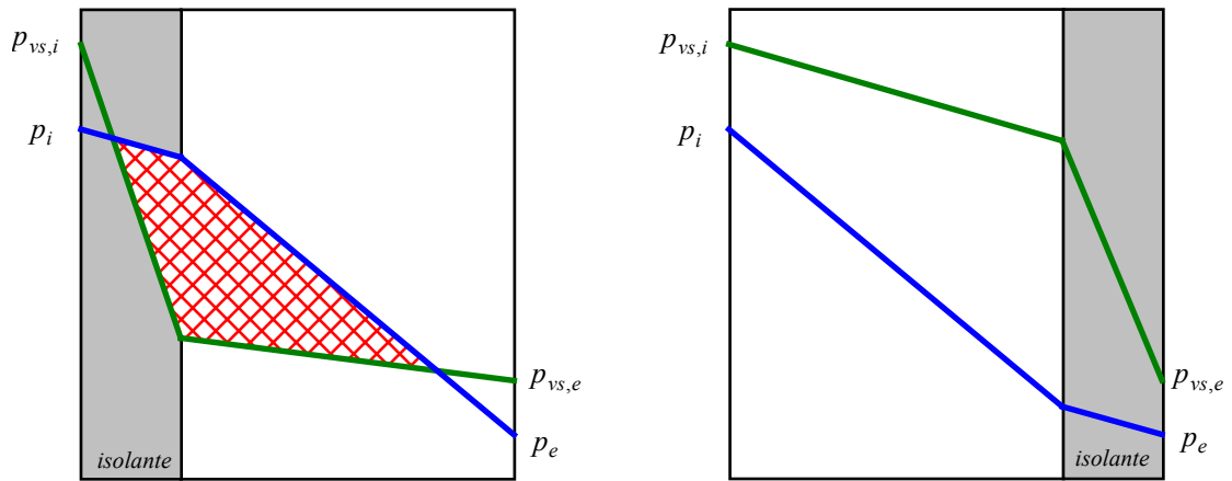
Figura 8. Effetto della disposizione degli strati sulla condensazione all'interno della parete.
