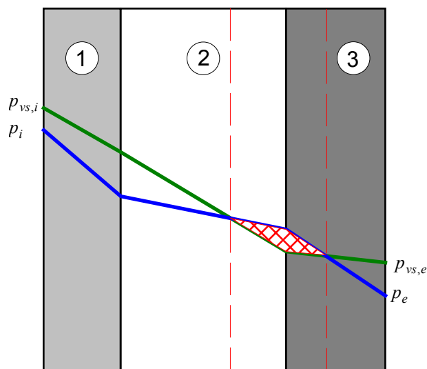
Figura 7. Condensazione in una zona all'interno della parete.
