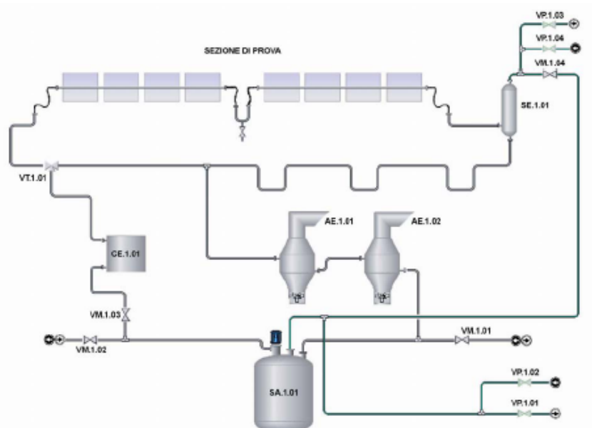
Fig. 31 - schema del circuito PCS
