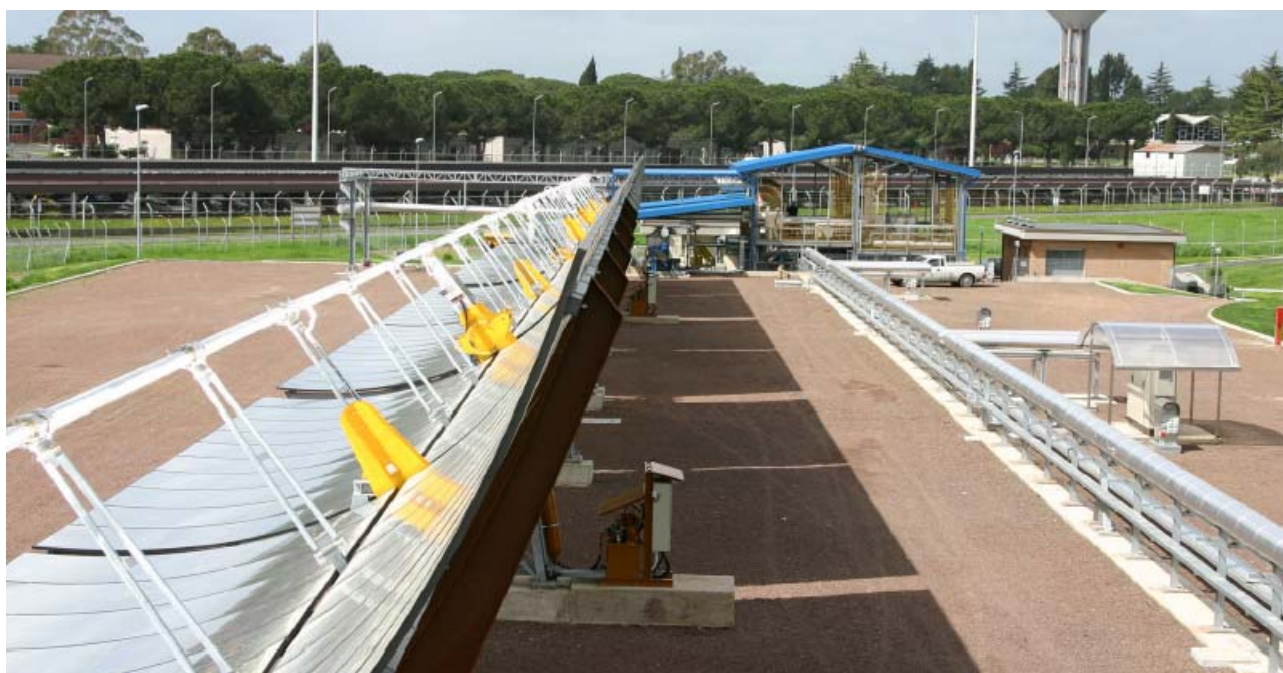
Fig. 30 - foto panoramica del circuito PCS con 2 collettori in prova
