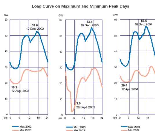
Fig. 12 - Diagrammi di carico della rete italiana nel 2003 [10] (nota: il 28 sett. 2003 avvenne il black-out generale)
