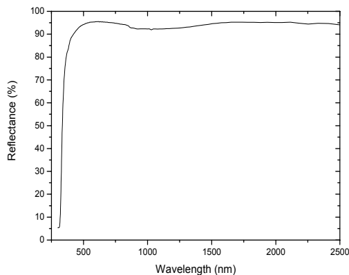
Fig. 28 – riflettanza misurata in funzione della lunghezza d'onda della radiazione solare.
