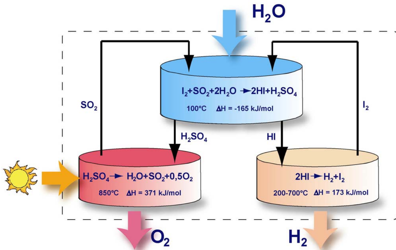
Fig. 41 - processo Zolfo-Iodio
