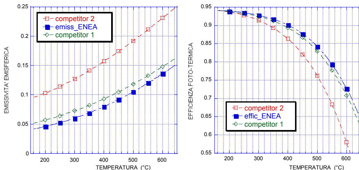
Fig. 26 – Emissività emisferica ed efficienza foto-termica misurate in laboratorio sui coating CERMET realizzati da ENEA e di 2 competitor commerciali.
