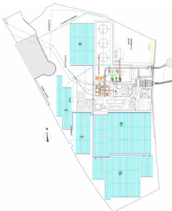
Fig. 39- Schema della disposizione dei collettori solari (in celeste) sull'area disponibile
