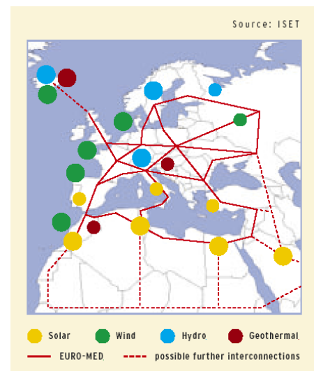
Fig. 3- schema esemplificativo dell'interconnessione elettrica euro-mediterranea (fonte ISET)
