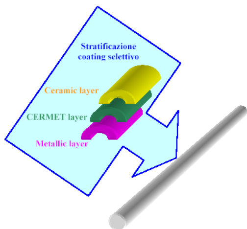
Fig. 24 - Schema del rivestimento selettivo a base di CERMET
