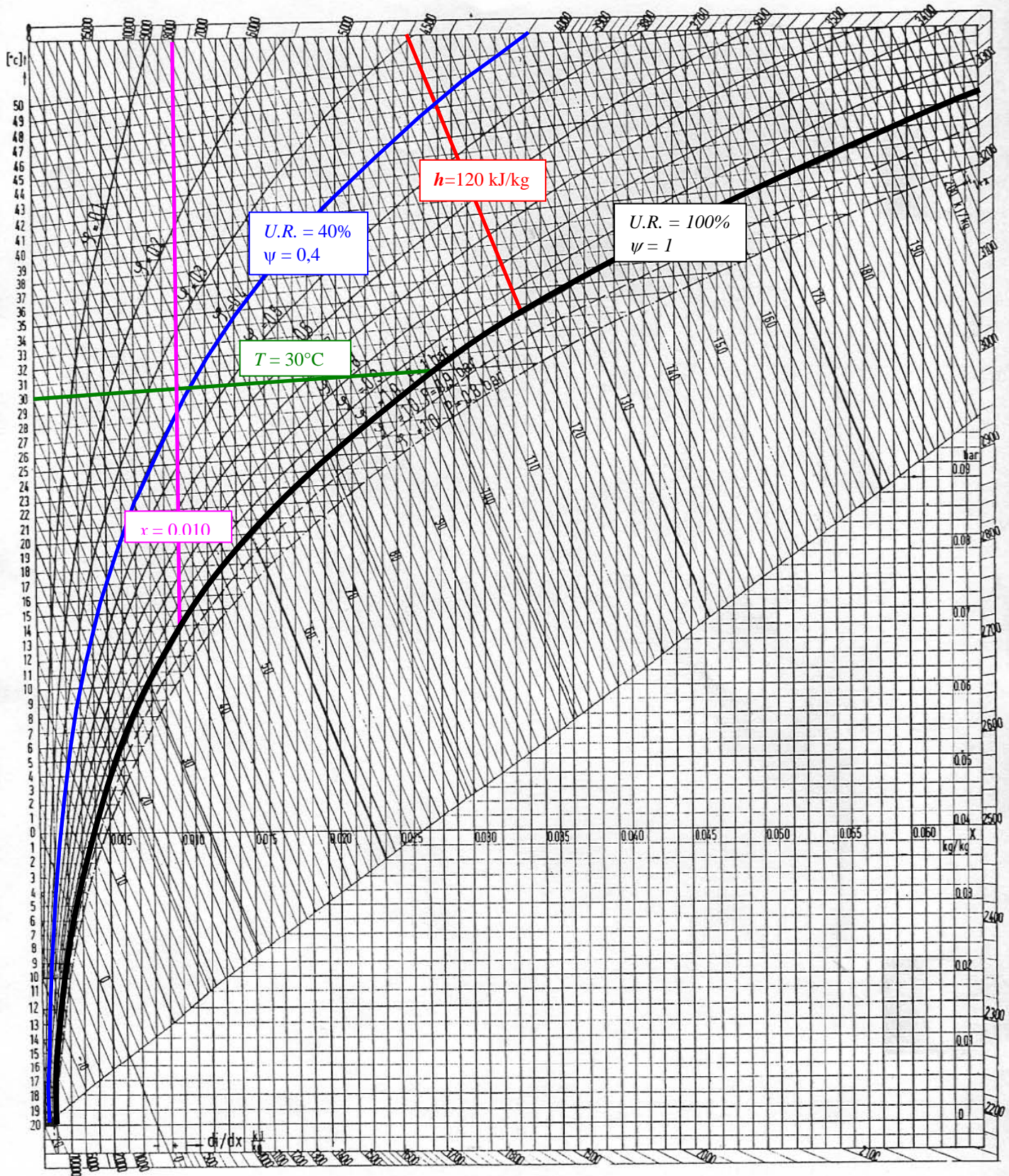
Diagramma di Mollier per l'aria umida (da -20^{\circ} a +50^{\circ}\text{C} ) i_{1+x} in \text{kJ/kg} , x in \text{kg/kg} .
