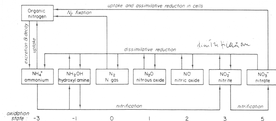
Fig. 4.6 - Trasformazioni dell'Azoto nei processi di nitrificazione e denitrificazione
