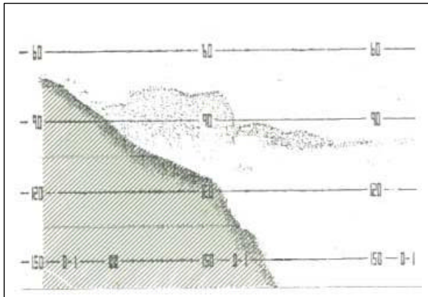
Fig. 6.5 – Deep Scattering Layer (DSL)
