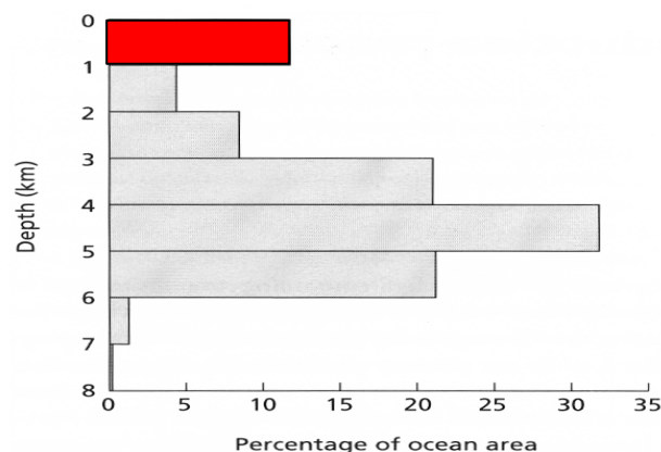
Fig. 2.1 - Proporzioni delle superfici oceaniche in relazione alla profondità. La profondità media è di 3.7 km. (Da Sunderman, 1986)
