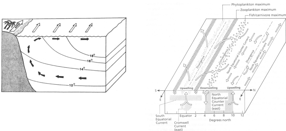
Fig. 3.5 - Schema di formazione di upwelling costieri e del largo.
