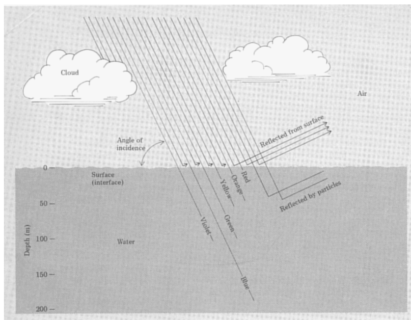
Fig. 3.1 - La penetrazione della luce nell'acqua nelle sue diverse componenti.
