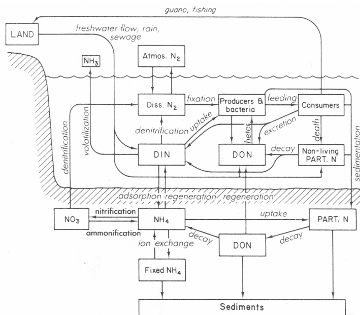
Fig. 4.7 - Ciclo semplificato delle principali trasformazioni e trasporti dell'Azoto in mare
